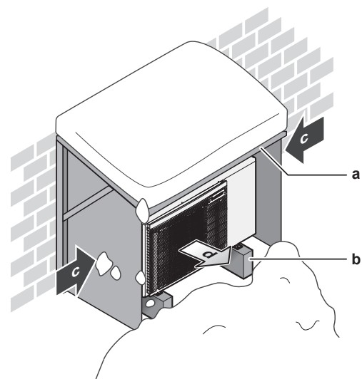
a Κάλυμμα ή στέγαστρο για προστασία από το χιόνι b Βάθρο
