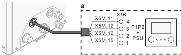
a Χειριστήριο: Απαιτείται για τον χειρισμό. Παρέχεται με τη μονάδα ως παρελκόμενο.
