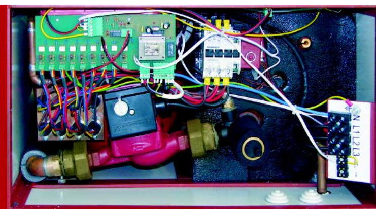
Ηλεκτρονικό κύκλωμα λέβητα
